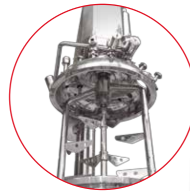
MCR. Equipo de mezcla con agitador contra-rotación y mixer. Preparación de productos de alta viscosidad a temperatura y presión controladas.
